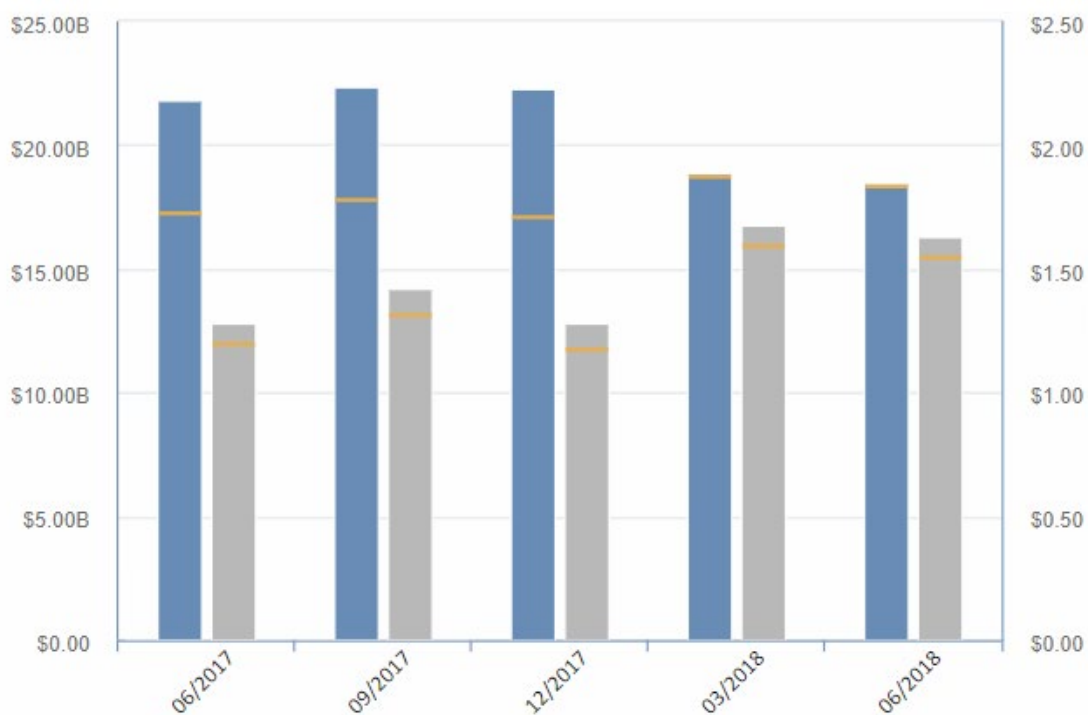
Рис. 1. График доходности Citigroup Inc.
